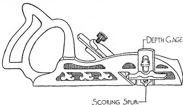
FIG. 66. RABBET OR REBATE PLANE.
